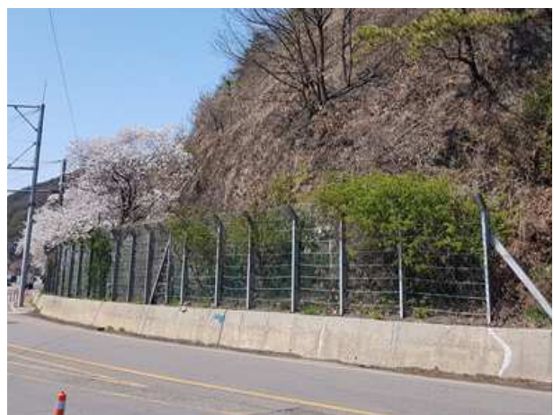
낙석방지울타리 전경
