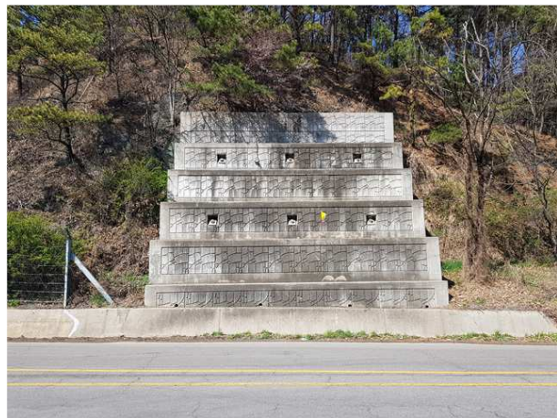
계단식 옹벽 전경
